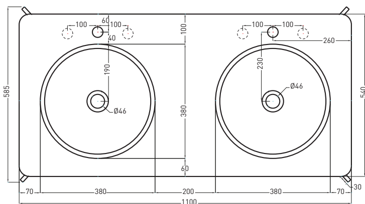
TOP
