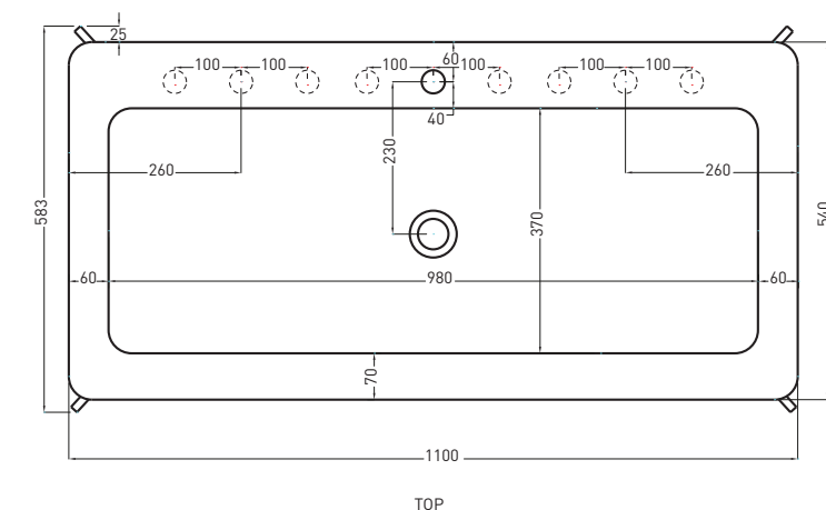
TOP
