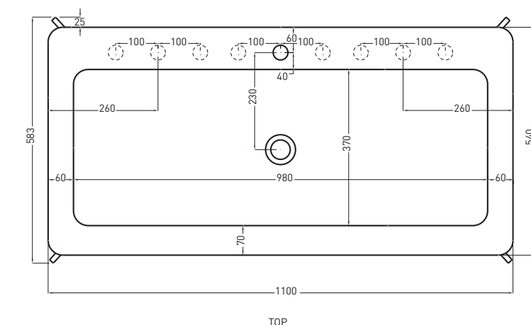
TOP
